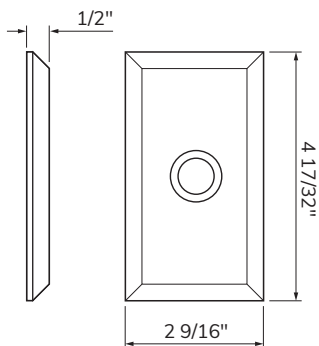
-G1 RECTANGLE
